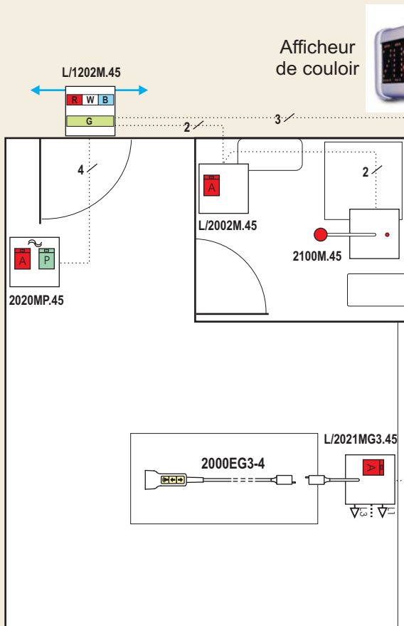
Ch. 1 lit + WC/douche/lavabo
