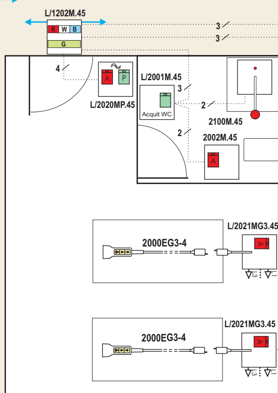
Ch. 2 lits + WC/douche
