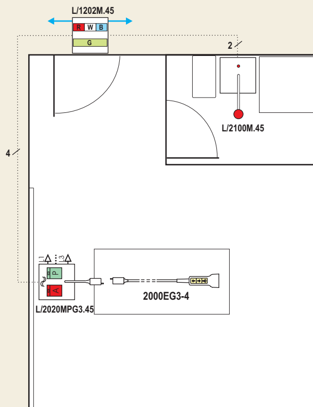
Ch. 1 lit + WC/douche
